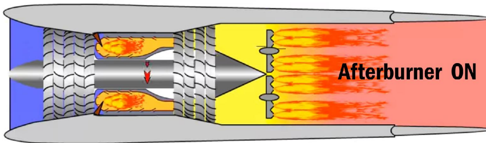
ስእሊ ቁ. 2 ዝተወልዐ አፍተርበርነር።
