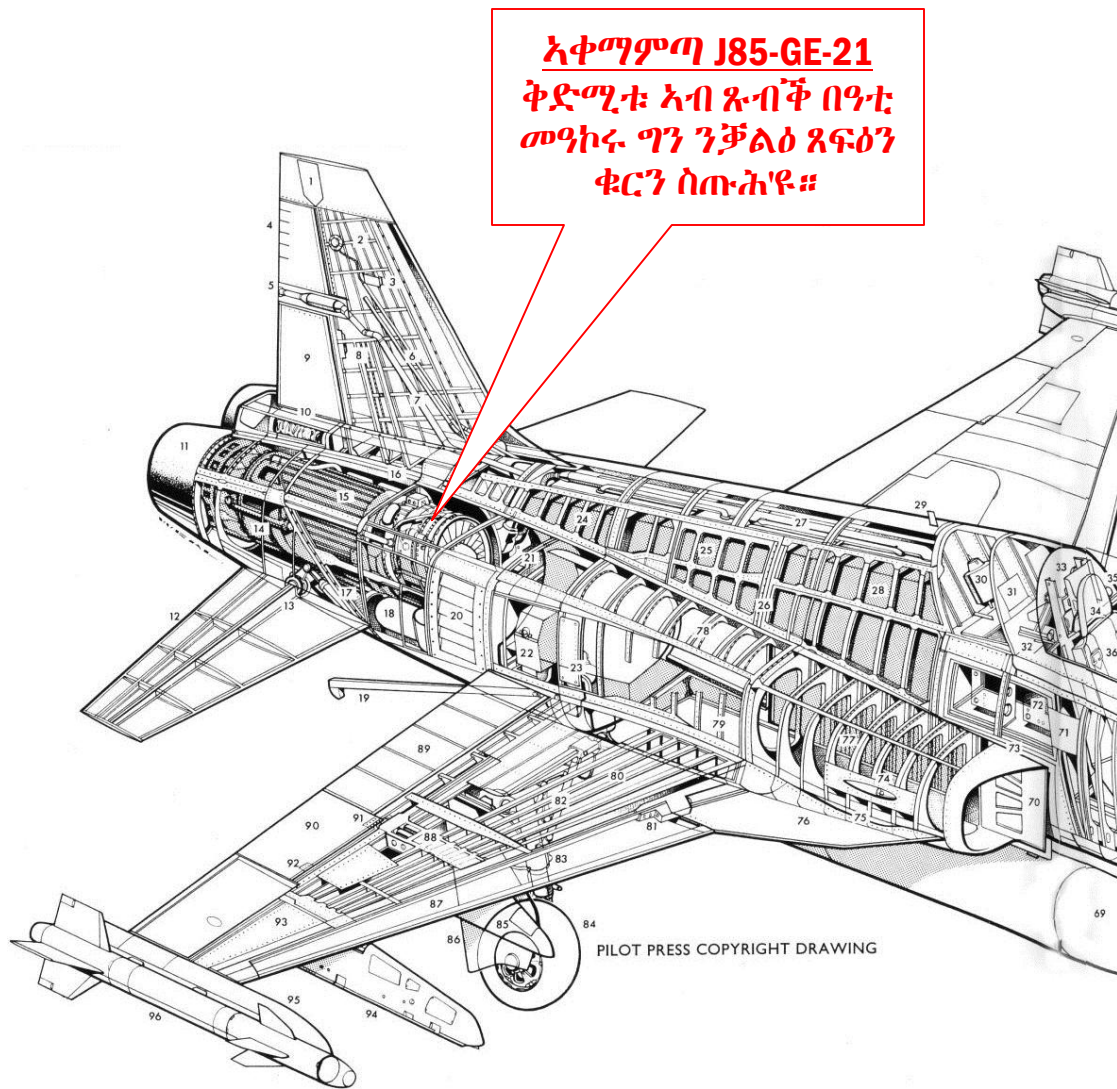
ፎቶ 30 አቀማምጣ J85-GE-21፡ አብ ውሽጢ ገንዲ ስብነት ናይ F-5E Tiger።
