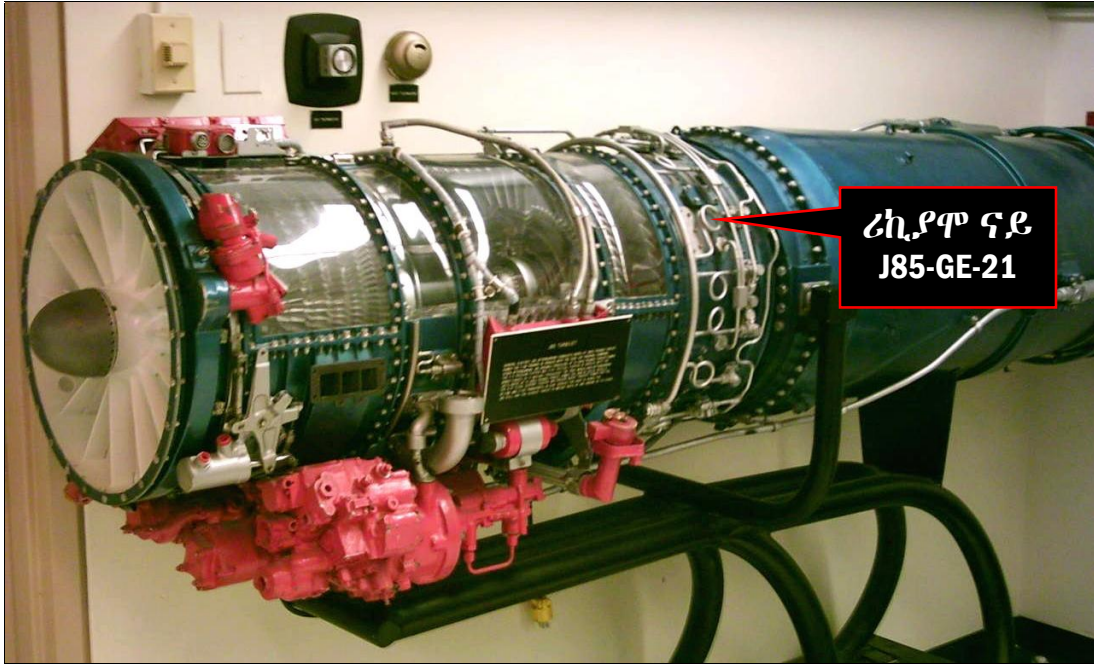
ፎቶ 22 ሪኬያሚ፡ ኣብ ቤተ መዘክር ናይ J85-GE-21። ሪኬያሚ፡ ንኣፍተርበርነር ጀት ፊወል ዝምግቡ ክባውያን ቱቦታት ኢዮም።
